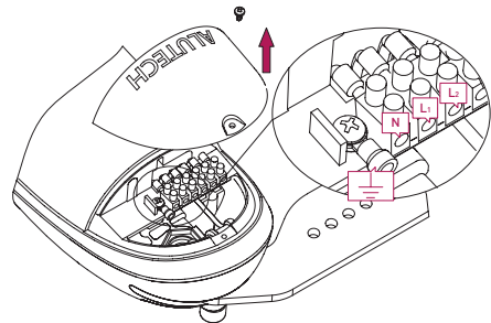
Малюнок 19. Підключення двигуна AM-5000 до модуля. Перемички XN1 і XN2 модуля повинні бути встановлені (контакти замкнені)!
