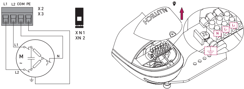
Рисунок 19. Подключение привода AM-5000 к модулю. Переключки XN1 и XN2 модуля должны быть установлены (контакты замкнуты)!
