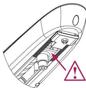
Рисунок 14. После монтажа привода не должно быть контакта вилки с корпусом
