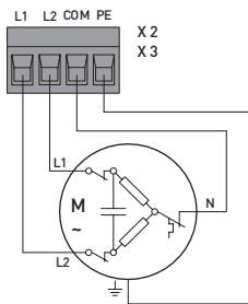
Малюнок 19. Підключення двигуна AM-5000 до модуля. Перемички XN1 і XN2 модуля повинні бути встановлені (контакти замкнені)!
