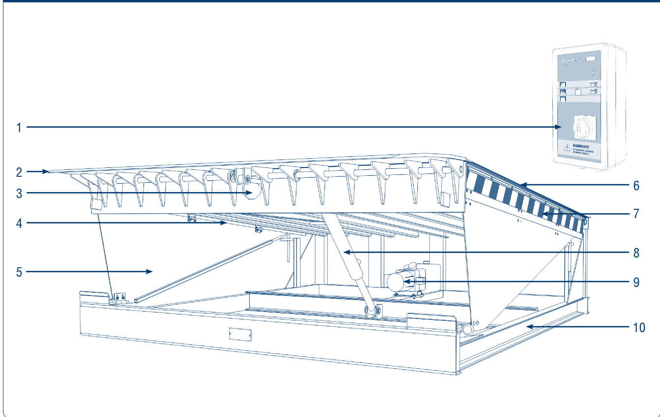
Рис. 5.2.1. Общий вид
